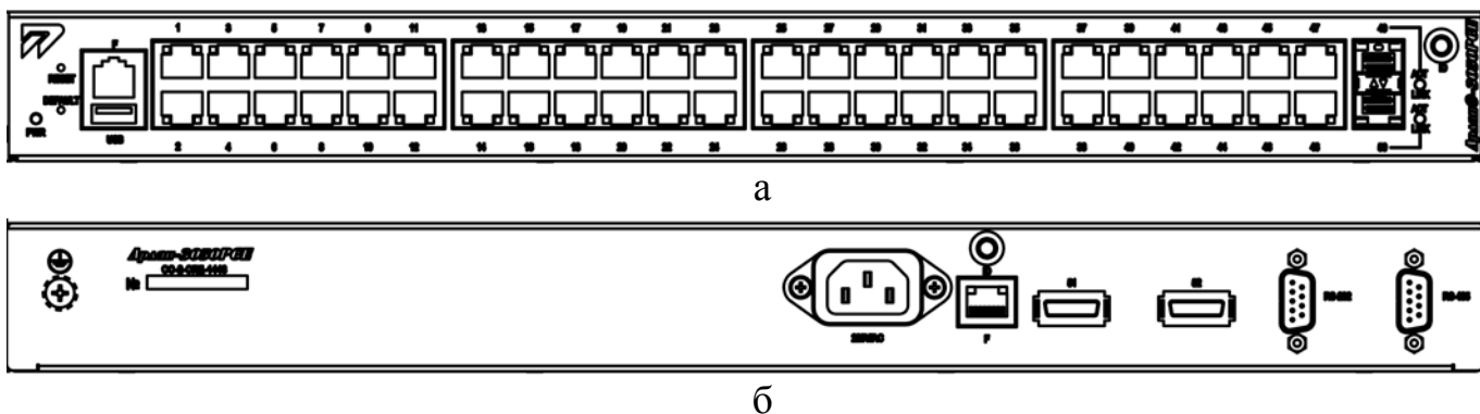
а – передняя панель; б – задняя панель.
