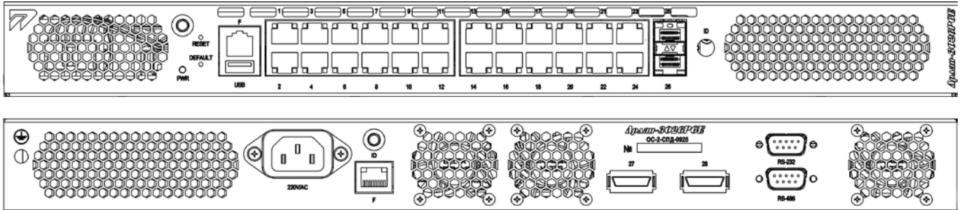
Рисунок Б.1 – Внешний вид лицевой и задней панелей коммутатора Арлан-3226GE/PGE(-S)
