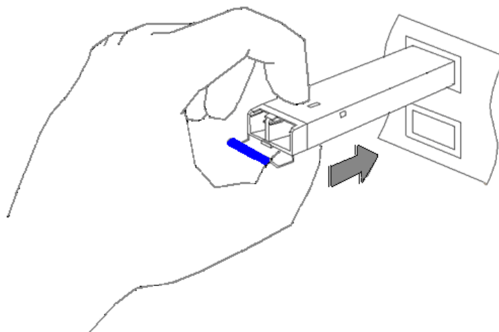
Рисунок 7 – Установка SFP-модуля в верхний разъем SFP
