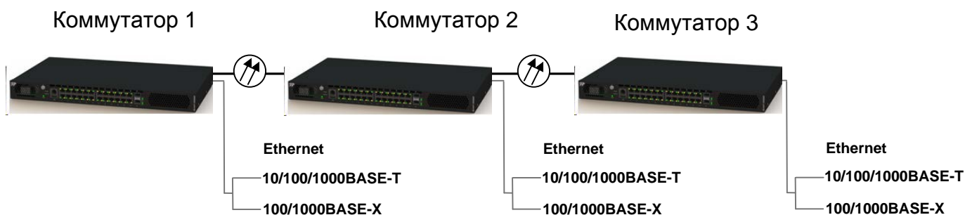
Рисунок 6 – Включение коммутаторов в линейную топологию
