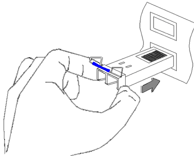
Рисунок 8 – Установка SFP-модуля в нижний разъем SFP
