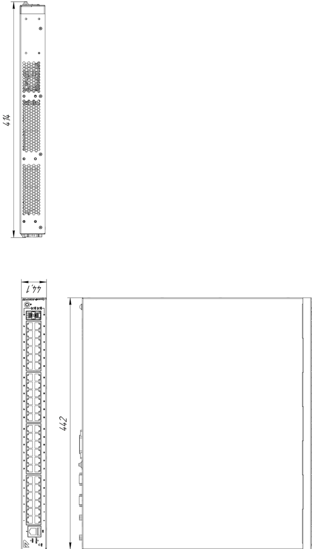
Рисунок А.2 – Габаритные и установочные размеры коммутатора Арлан-3250GE/PGE(-S)
