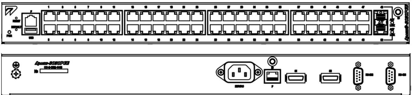
Рисунок Б.2 – Внешний вид лицевой и задней панелей коммутатора Арлан-3250GE/PGE(-S)
