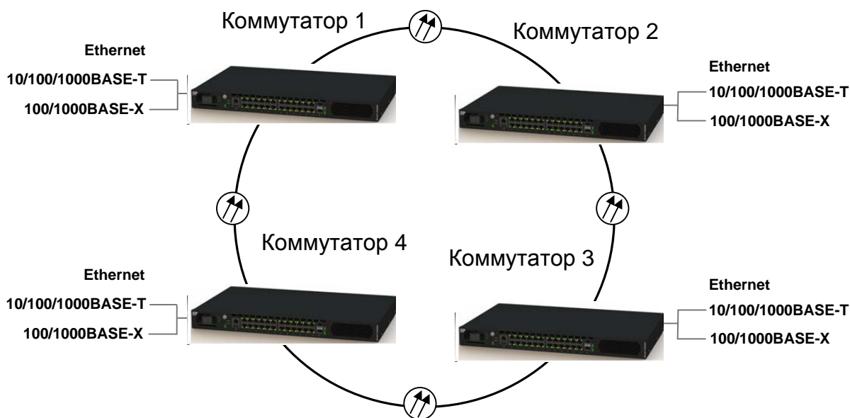
Рисунок 5 – Включение коммутаторов в кольцевую топологию
