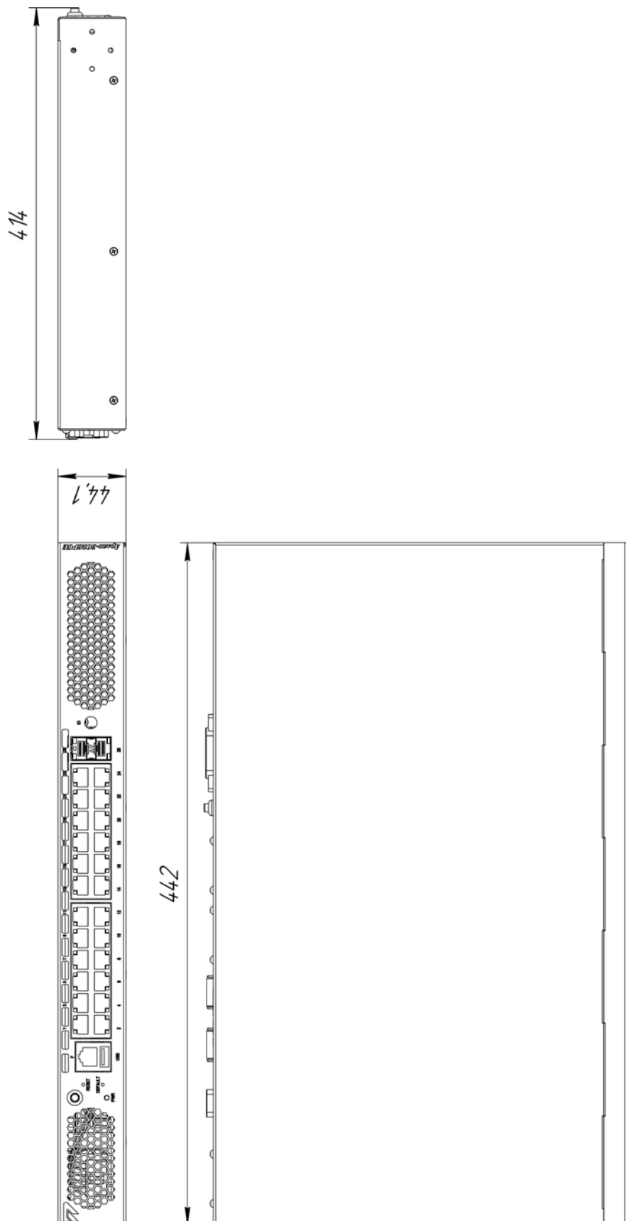
Рисунок А.1 – Габаритные и установочные размеры коммутатора Арлан-3226GE/PGE(-S)
